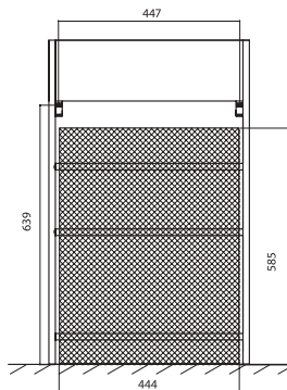
Тумба Sogno (3 полки)
