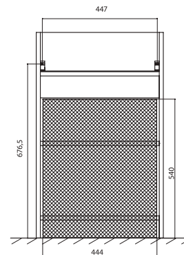
Тумба Sogno (1 дверь)
