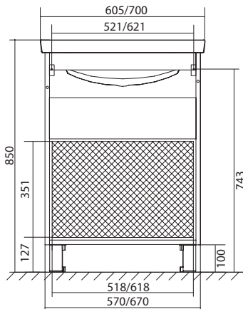
Тумба NEW Aris
