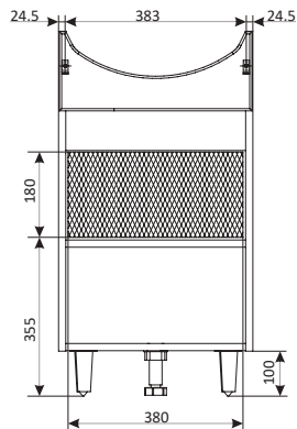
Тумба NEW Aris
